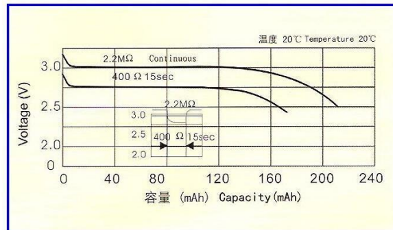
脉冲放电曲线
