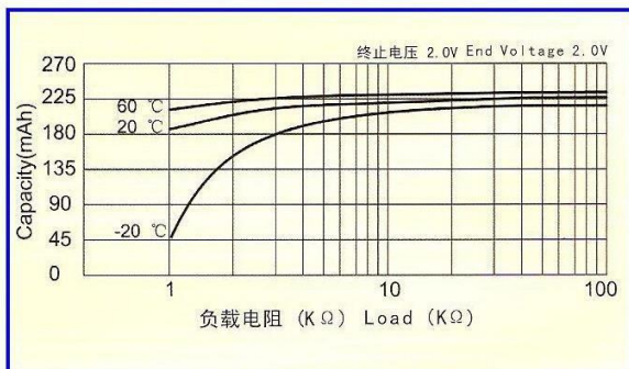
电阻容量曲线
